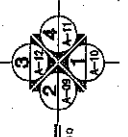
แปลนฐานราก มาตรฐาน 1 : 40
